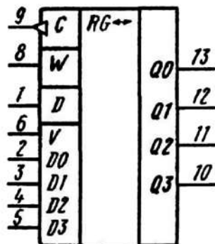
Условное графическое обозначение К533ИР16, КН533ИР16
