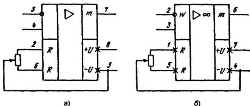
Схемы балансировки K140УД8 (а) и КР140УД8 (б)
