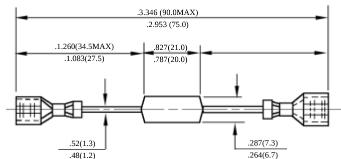
外形尺寸 Outline dimensions
